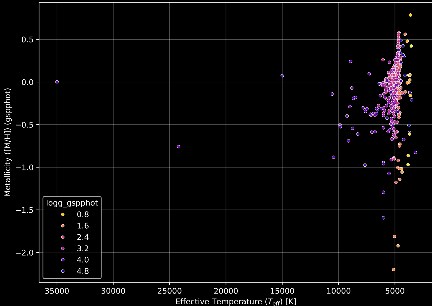
APOGEE DR17 Field: [030+08] Stellar Population Parameters (n= 596)
